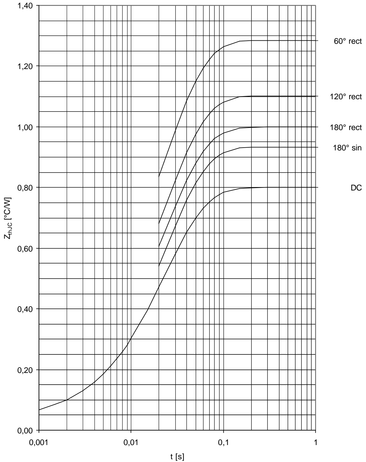
Transienter innerer Wärmewiderstand Gleichrichter / Transient thermal impedance rectifier Z_{thJC} = f(t) Parameter: Stromflußwinkel / Current conduction angle Q
